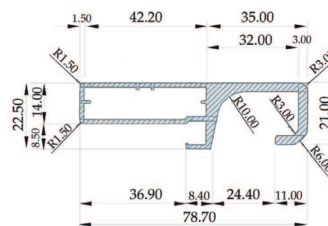
FG786 Aluminum Profile for Door โปรไฟล์อลูมิเนียม
