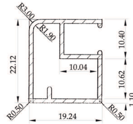
FG104 Aluminum Profile for Door โปรไฟล์อลูมิเนียม
