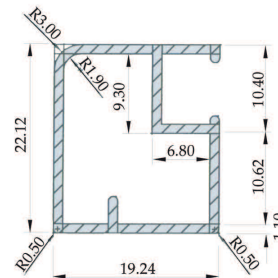
FG787 Aluminum Profile for Door โปรไฟล์อลูมิเนียม
