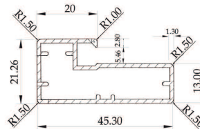
FG105 Aluminum Profile for Door โปรไฟล์อลูมิเนียม
