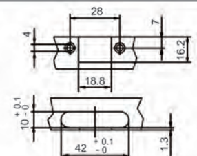
ระยะเจาะบนเฟรมอลูมิเนียม Drilling dimensions on aluminium frame
