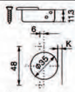
Hinge cup types แบบของถ้วยบานพับ
