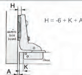
บานในขอบ Inset
