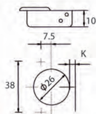
Hinge cup types แบบของถ้วยบานพับ
