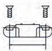
ระยะเจาะบนเฟรมอลูมิเนียม Drilling dimensions on aluminium frame
