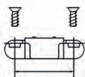
ระยะเจาะบนเฟรมอลูมิเนียม Drilling dimensions on aluminium frame
