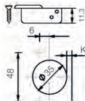
MS001+MS002 อุปกรณ์ยึดล็อกหน้าบาน push open latch/ door holder
