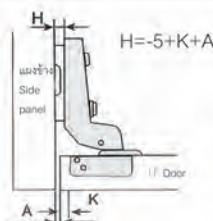
ทับครึ่งขอบ Half Overlay
