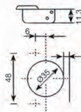
Hinge cup types แบบช่องถ้วยบานพับ
