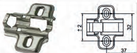
Mounting Plate Height: 2 mm. / ความสูงฐานบานพับ: 2 มม.
