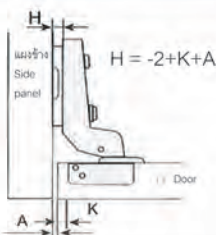
ทับครึ่งขอบ Half Overlay
