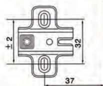
Mounting Plate Height: 3 mm. / ความสูงฐานบานพับ: 3 มม.
