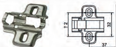
Mounting Plate Height: 0 mm / ความสูงฐานบานพับ: 0 มม.
