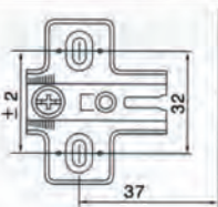
Mounting Plate Height: 2 mm. / ความสูงฐานบานพับ: 2 มม.
