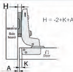
บานในขอบ Inset
