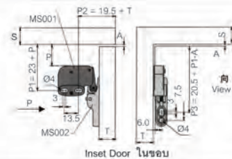
Inset Door ในขอบ
