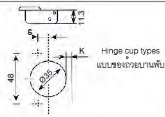
บานในขอบ Inset
