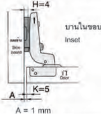
ทับครึ่งขอบ Half Overlay
