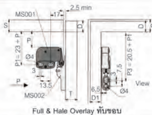
Full & Half Overlay ทับขอบ
