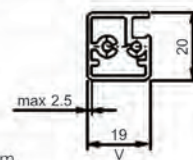
ระยะเจาะบนเฟรมอลูมิเนียม Drilling dimensions on aluminium frame
