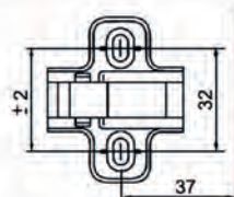
Mounting Plate Height: 2 mm. / ความสูงฐานบานพับ: 2 มม.
