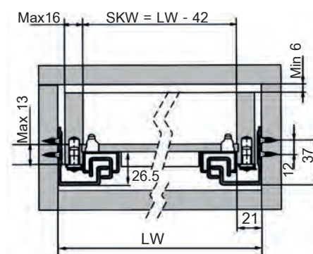
Standard drawer ลิ้นชักมาตรฐาน
