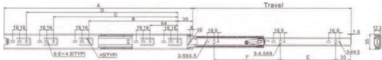
ขนาดของรางลิ้นชัก
