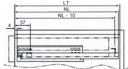
Inner drawer ลิ้นชักด้านใน
