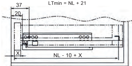
Inner drawer ลิ้นชักด้านใน
