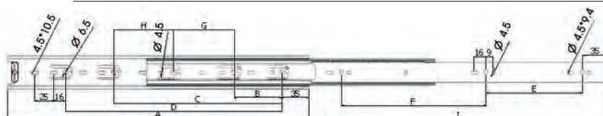
ขนาดของรางลิ้นชัก
