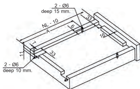
Drawer size and boring ขนาดลิ้นชักและรูเจาะ
