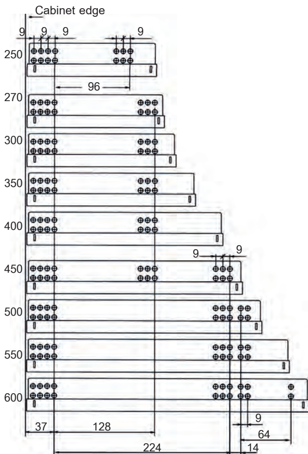
Drawer size and boring ขนาดลิ้นชักและรูเจาะ
