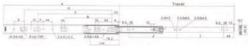
ขนาดของรางลิ้นชัก
