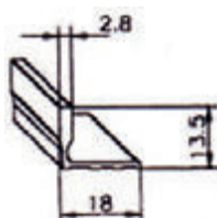
Lower rail 3 meters / รางอลูมิเนียมล่าง
