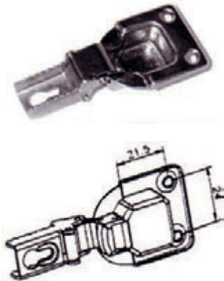
Concealed hinge / บานพับซ่อน
